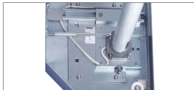
Sistema de desplaçament horitzontal per a l'eix.
